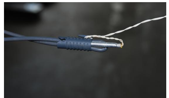
Gegen Herausziehen gesichertes Zündkabel einer elektrischen Sprengkapsel
