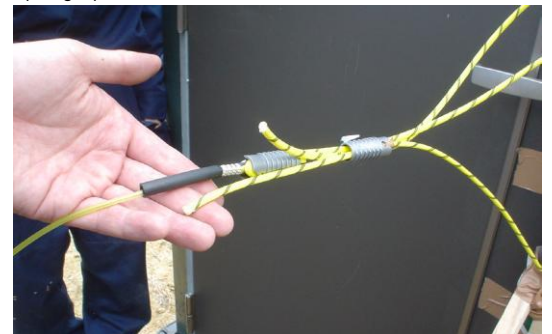
Zündkette mit Shock Tube - Auslösung
